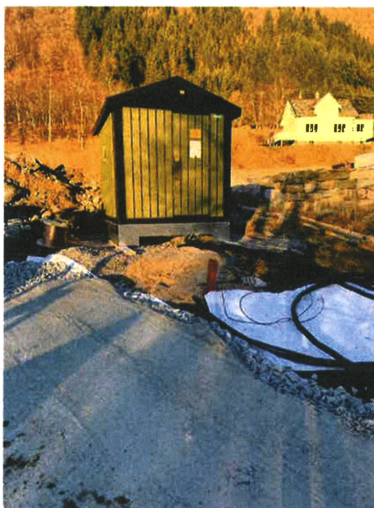
Mosvold 4. Siemens nettstasjon med 315 kVA trafo er satt i drift. Erstatte trafo i mast.
