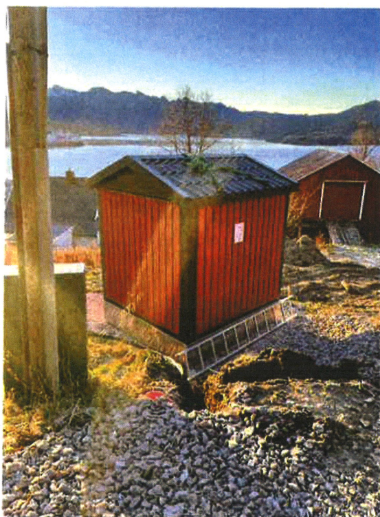
Mosvold Koblingskiosk. Knutepunkt for Ørnes 2 og fjellinja.
