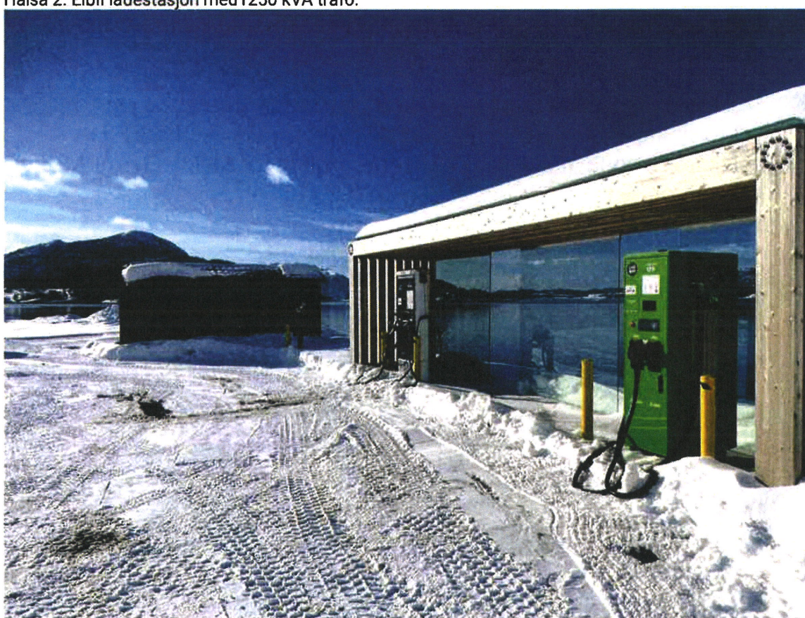
Ørnes 6. Elbil ladestasjon med 1250 kVA trafo.
