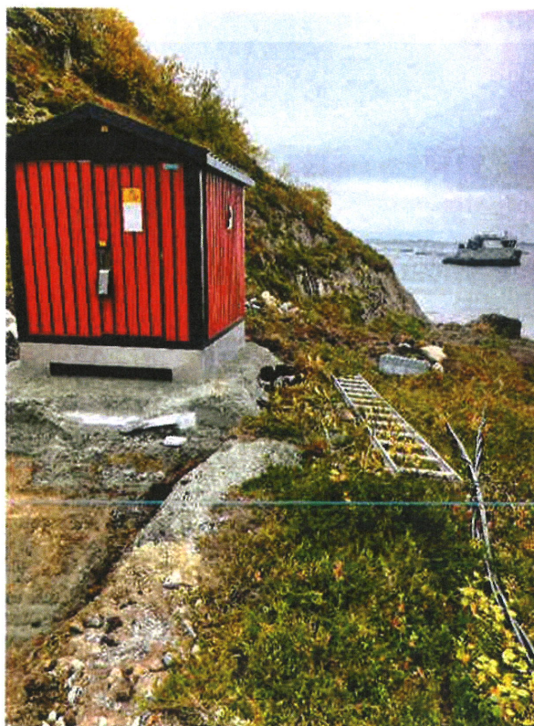
Åmøyhamn 4. Siemens nettstasjon med 315 kVA trafo er satt i drift til Norcod.
